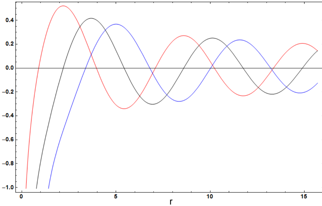
Neumann Funktionen
