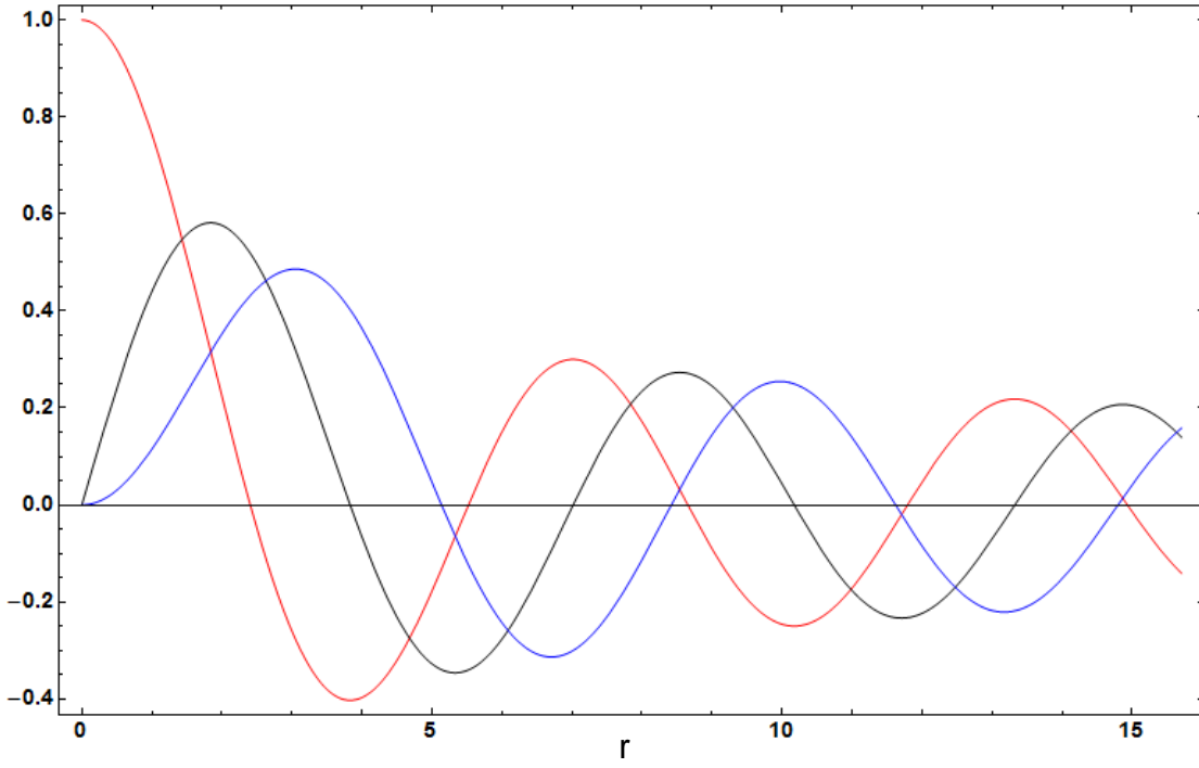
Bessel Funktionen
